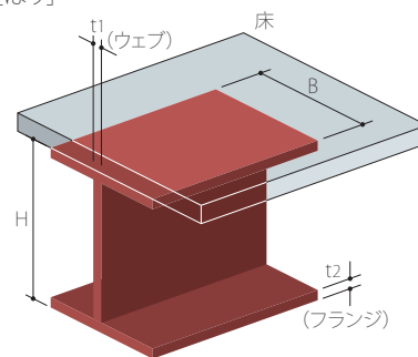
[はり]
