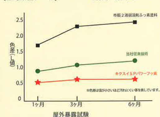
[低汚染性データ]
